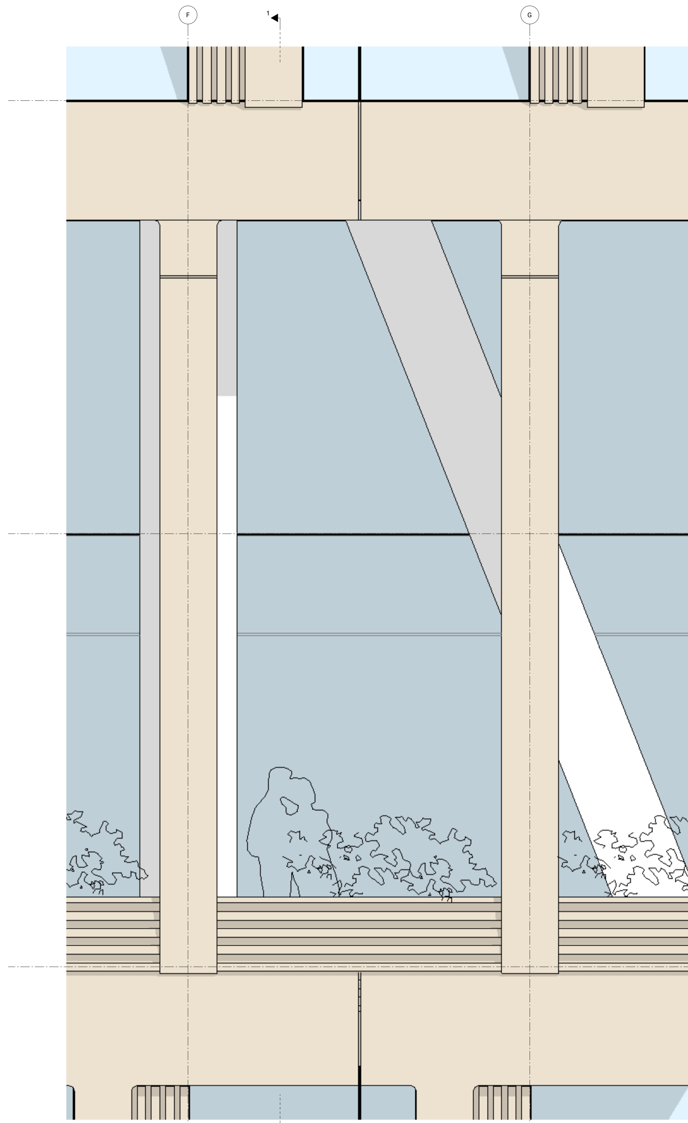
ELEVATION 1:20
